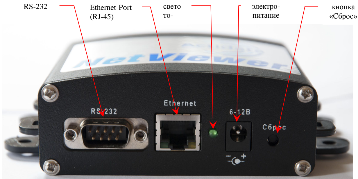
Рисунок 2. Вид разъемов на передней стороне контроллера Actidata NV1.1G
