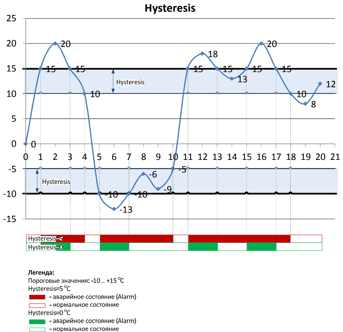
Рисунок 29. Графическое представление понятия Hysteresis
