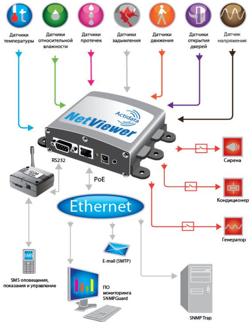
Рисунок 4. Схема работы Actidata NV1.1G
