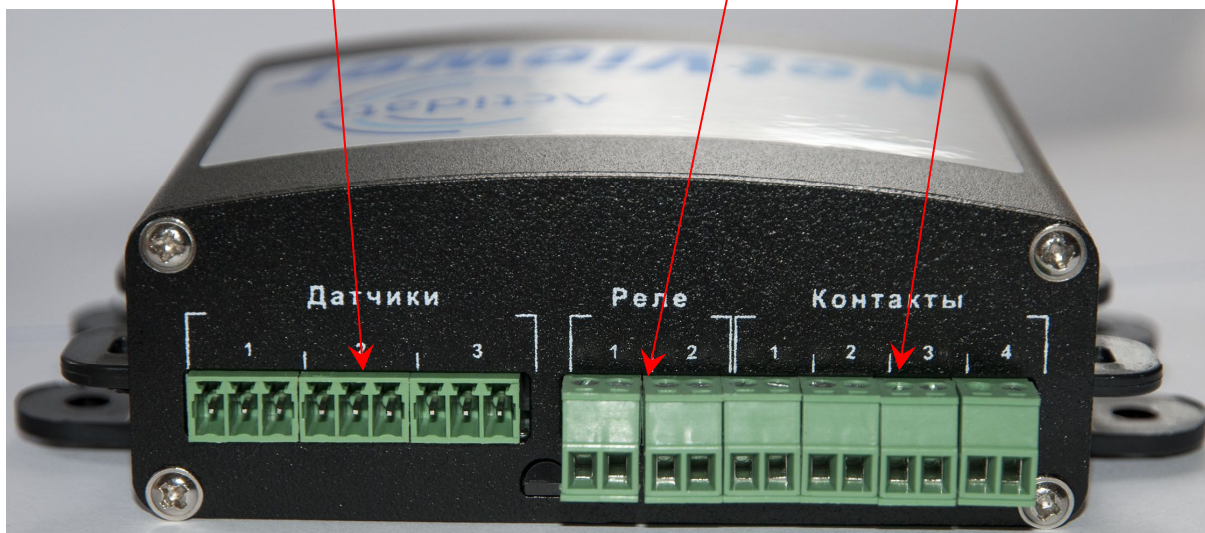
Рисунок 3. Вид разъемов с обратной стороны модели контроллера Actidata NV1.1G
