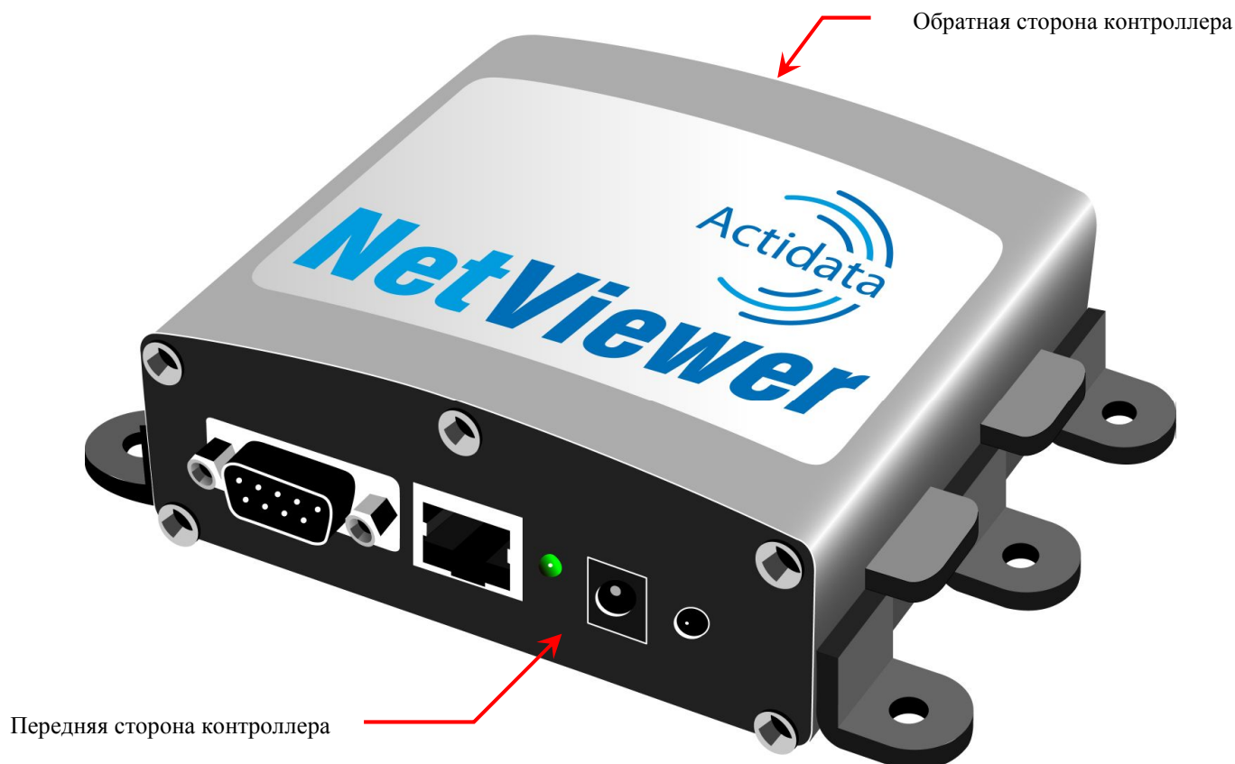
Рисунок 1. Внешний вид контроллера Actidata NV1.1G
