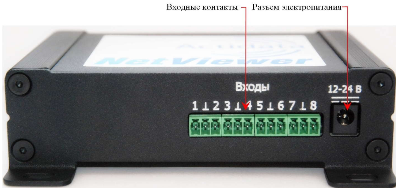
Рисунок 3. Вид разъемов с обратной стороны модели контроллера Actidata NV2
