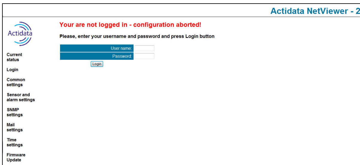
Рисунок 18. Отсутствие аутентификации
