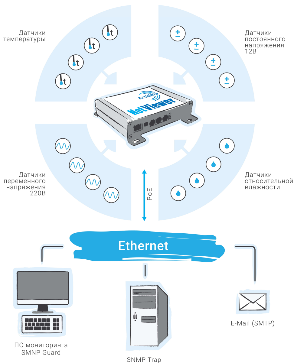
Рисунок 4. Схема работы Actidata NV2
